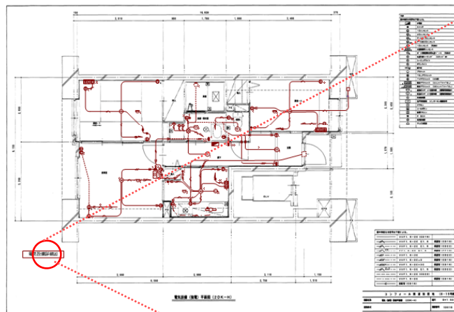
管理図(2)電気設備
