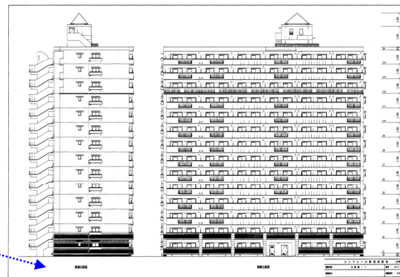
立面図-1
