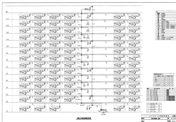
自動火災報知設備系統図
