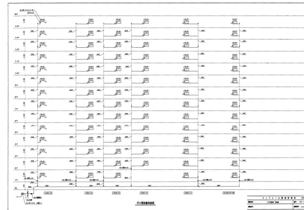
ガス管設備系統図
