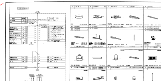
分電盤結線図・照明器具姿図
